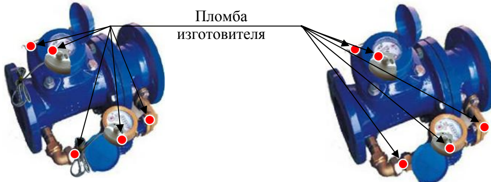
Рисунок 5 – Общий вид счетчиков исполнений Пульсар КХ 1 -И 1) , Пульсар ТХХ 1 -RS-485 1) и схема пломбировки
