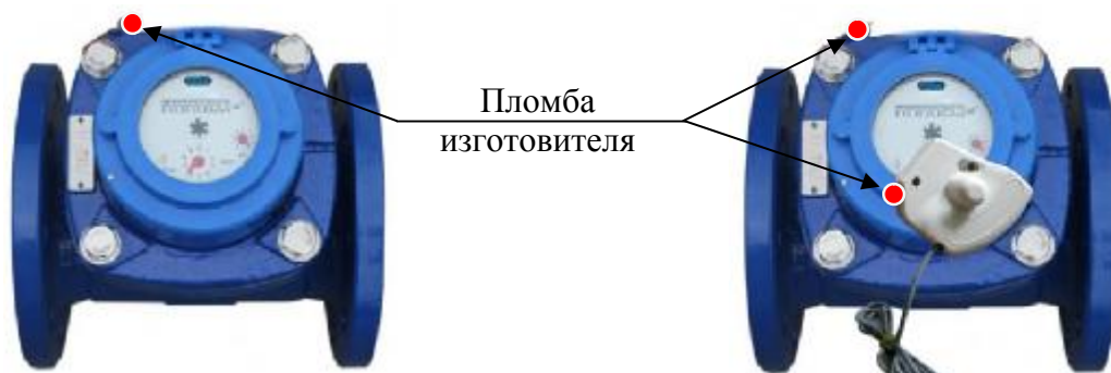
Рисунок 2 – Общий вид счетчиков исполнений Пульсар ТХХ 1 -И 1) , Пульсар ТХХ 1 -RS-485 1) , Пульсар ТГХ 1 -И 1) , Пульсар ТГХ 1 -RS-485 1) и схема пломбировки
