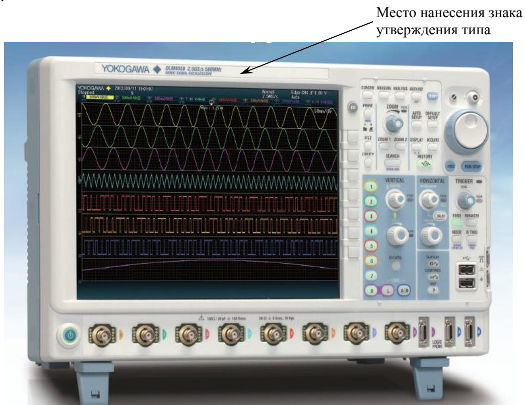
Рисунок 1. Общий вид и место нанесения знака утверждения типа на осциллографы цифровые DLM4038, DLM4058
