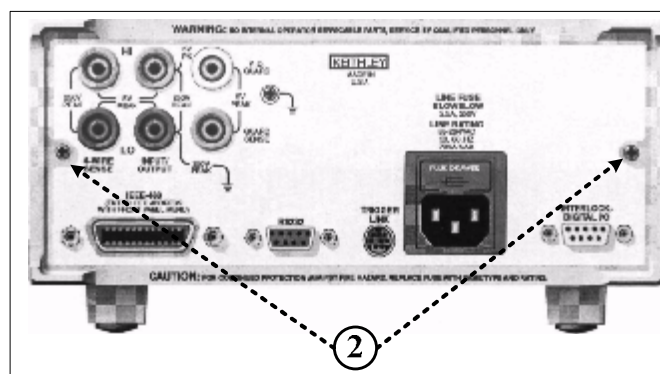
Примечание: ② - места пломбировки от несанкционированного доступа. Рисунок 6 – Калибраторы/мультиметры (модели 2400, 2410, 2430). Вид сзади
