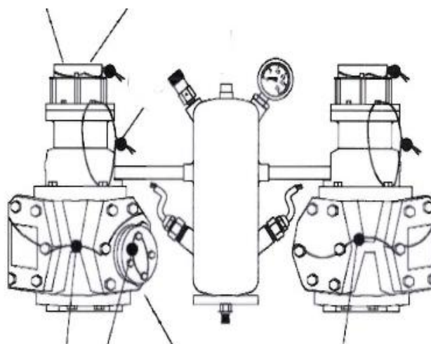
Р и с у н о к 2 – Схема пломбировки «PRIMA» фирмы «2A Mühendislik A.Ş.», Турция.
