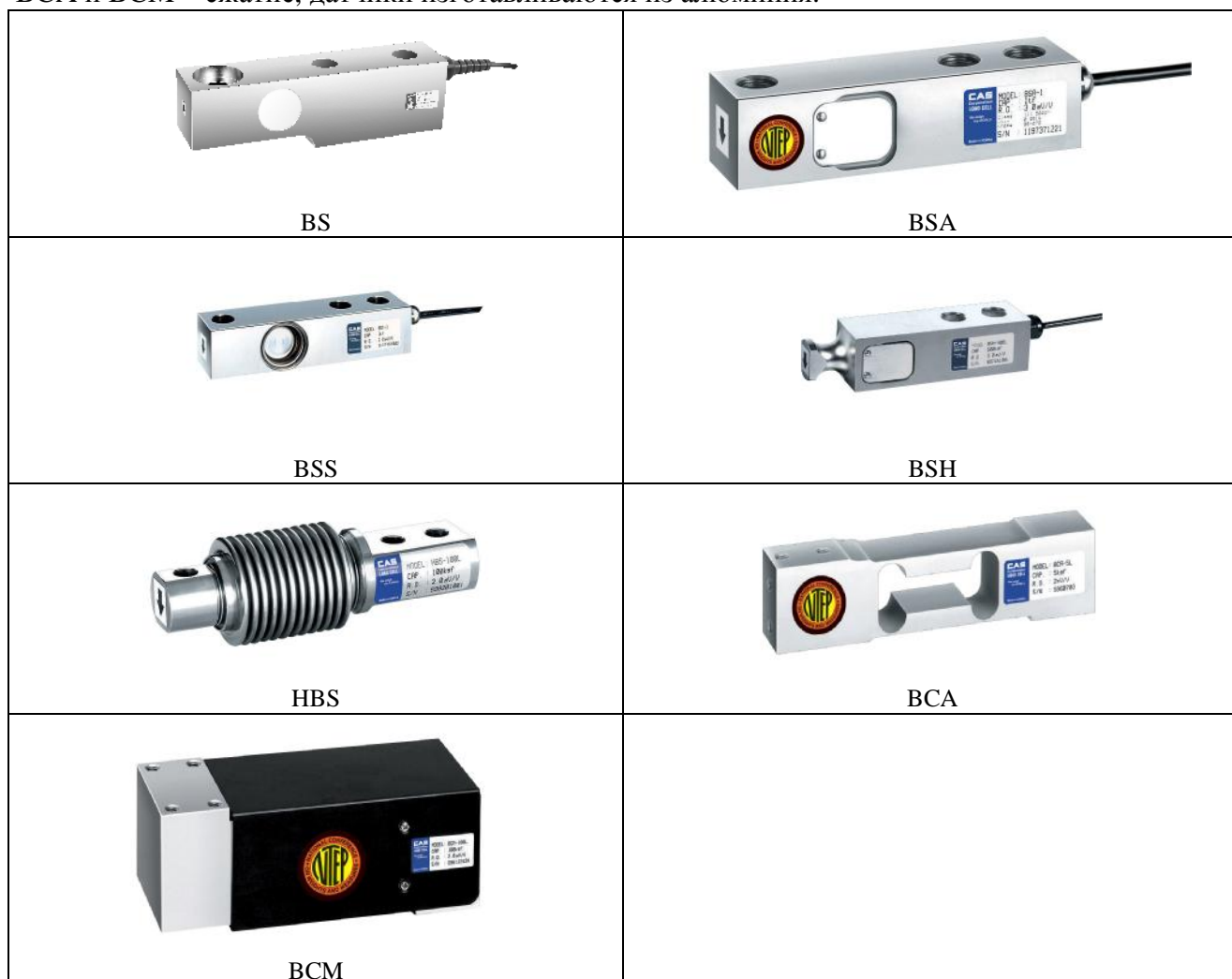
Рисунок 1 – Общий вид датчиков BS, BSA, BSS, BSH, HBS, BCA и BCM
