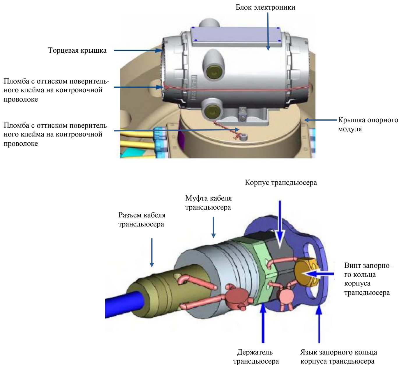
Рис. 2 - Места нанесения оттисков поверительных клейм на УПР
