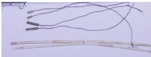
Рисунок 2 – Термометры ПТСВ-2К
