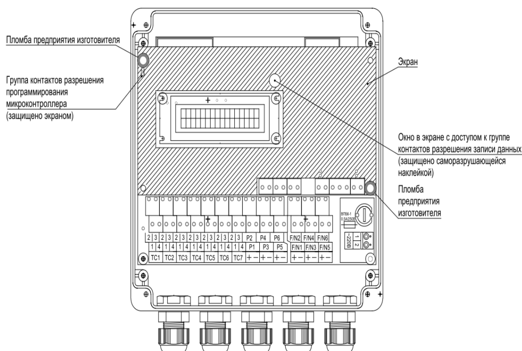
Рис 2. Схема пломбировки ТЭМ-106-1
