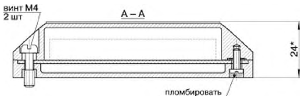
Рисунок 6 - Схема пломбировки генератора-преобразователя от несанкционированного доступа
