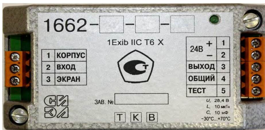
Рисунок 2 - Внешний вид генераторов-преобразователей СИЭЛ-1662
