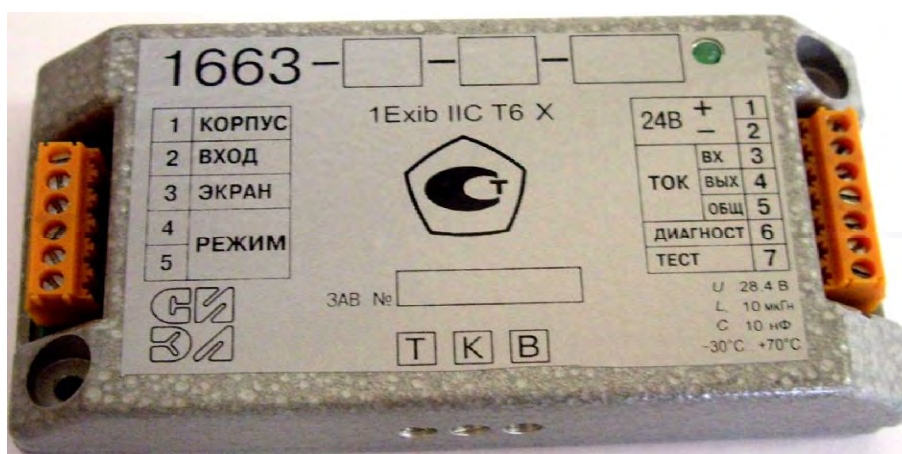
Рисунок 3 - Внешний вид генераторов-преобразователей СИЭЛ-1663
