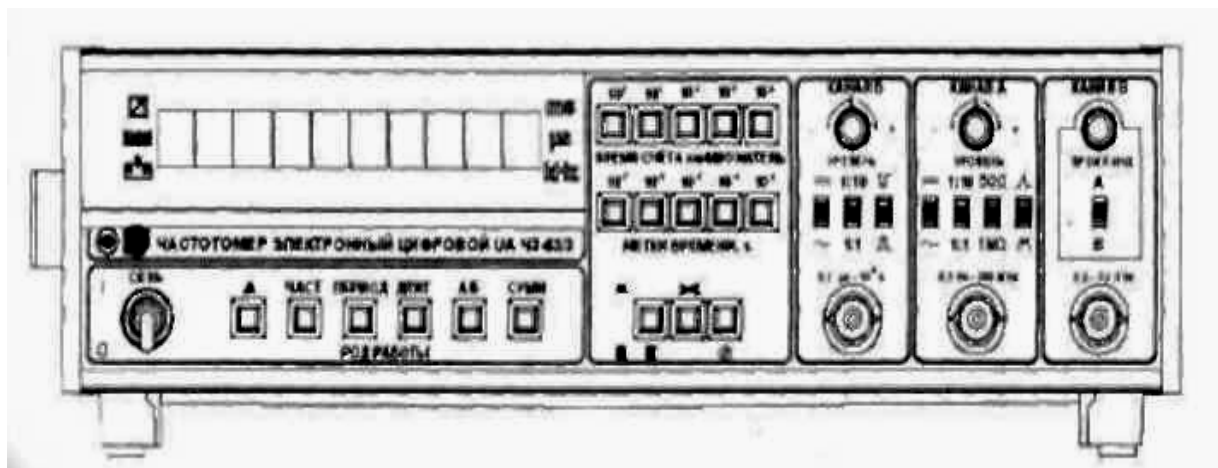
Рисунок 1.1 – Внешний вид передней панели частотомера УА ЧЗ-63/3
