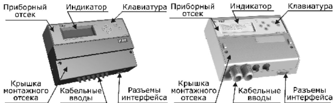
Рисунок 1 – Внешний вид тепловычислителя
