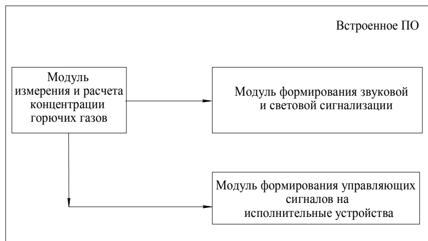
Рисунок 3 – Структура ПО
