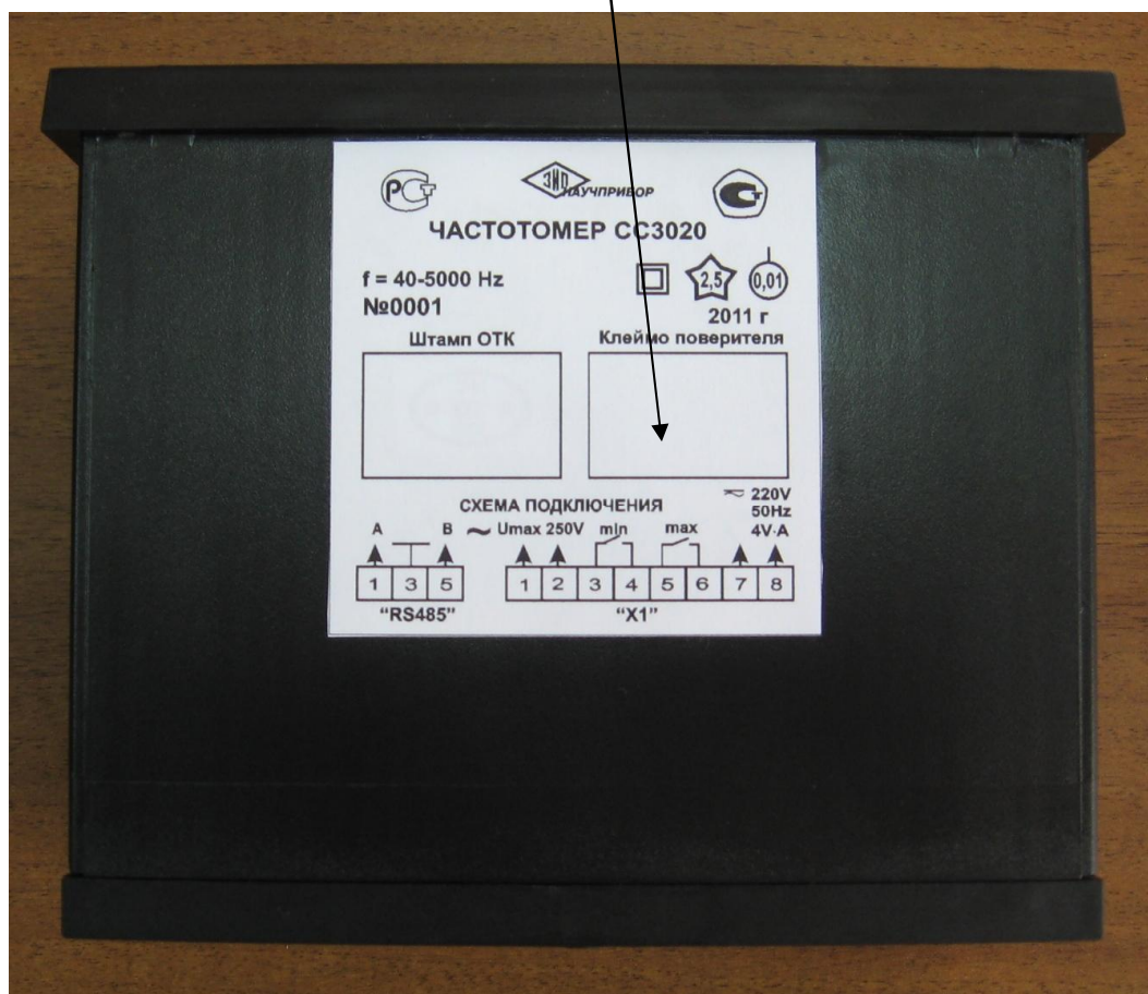
Рисунок 3. Место нанесения поверительного клейма
