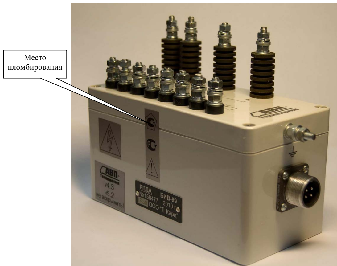
Общий вид блока измерения высоковольтного БИВ-89
